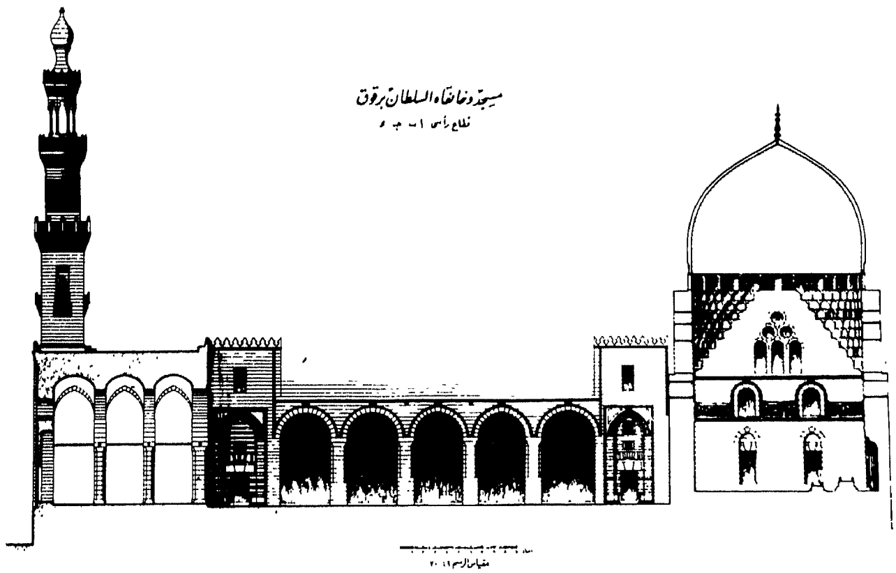
شكل ( ٥ ) يبين قطاع رأسى للمدرسة البرقوقية بقرافة المالك
